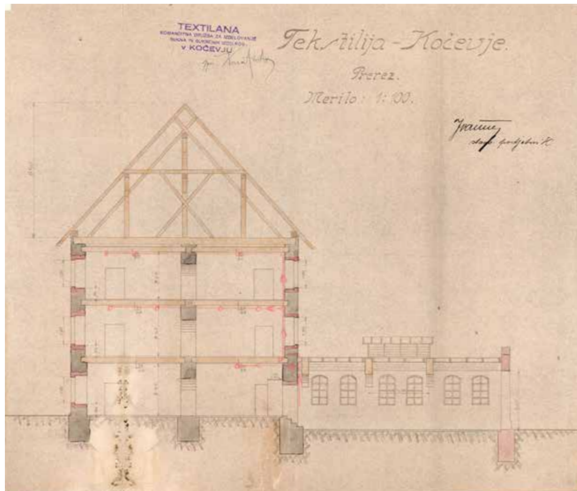
Prerez tovarniškega poslopja Textilane, komanditne družbe, okoli 1922
