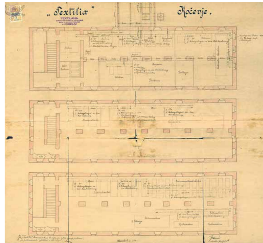
Prerez tovarniškega poslopja Textilane, komanditne družbe, okoli 1922
